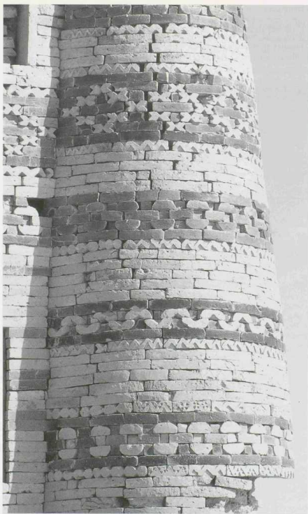
Abbildung 2: Früher Baudekor aus glasierten Ziegeln und Formziegeln an einem der ins 14. Jh. datierenden Adheri-Gräber, NW-Pakistan.
